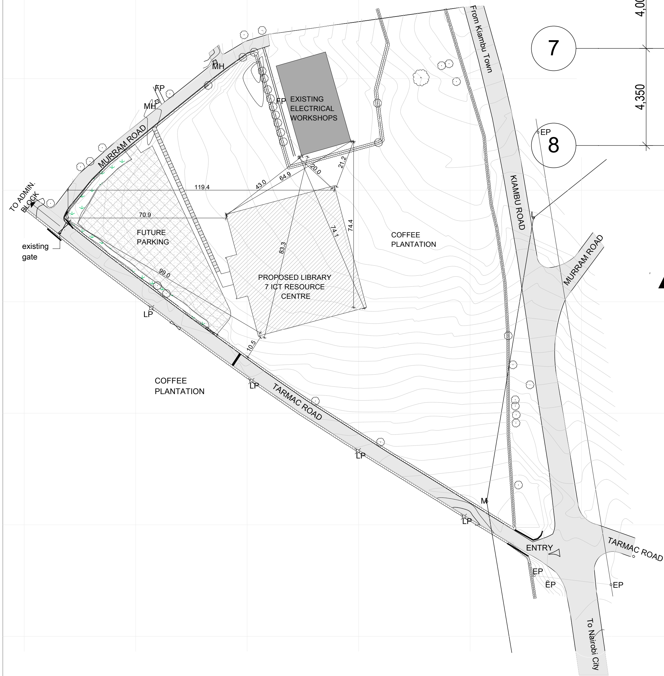
SITE LAYOUT 1:1000
